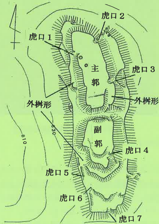
茶臼山城跡略測図 (1:2,000)
